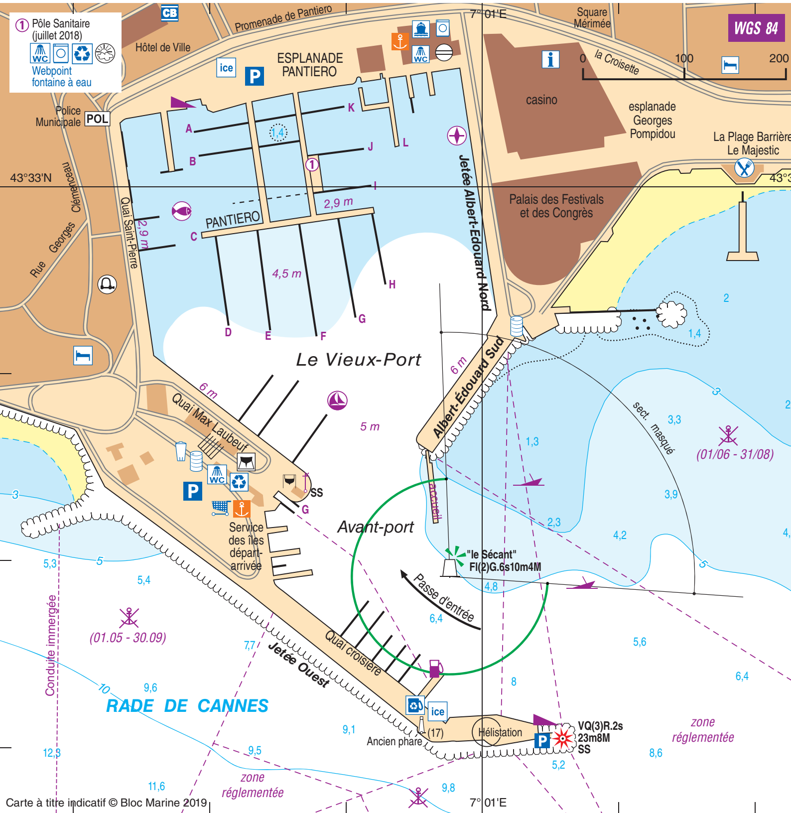
Plan bloc marine du Vieux Port de Cannes
